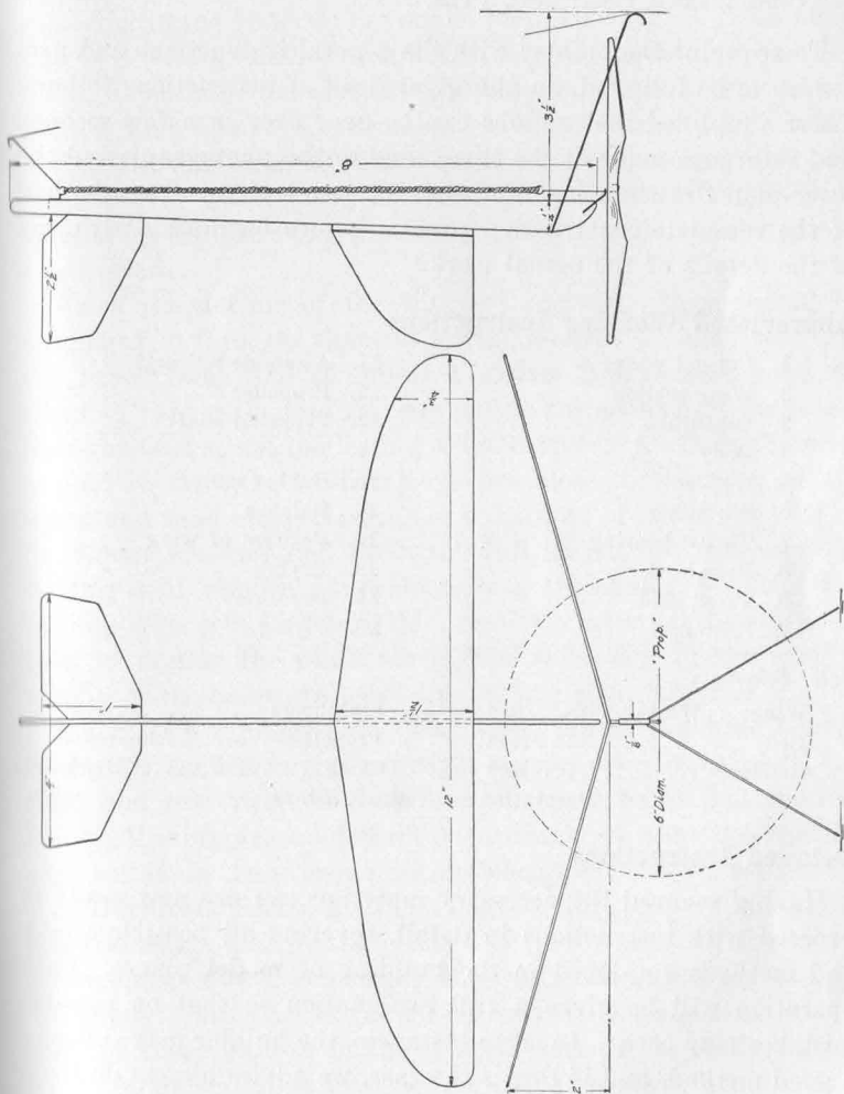
Fig. 71—3-Plan Drawing Junior Indoor Flyer
