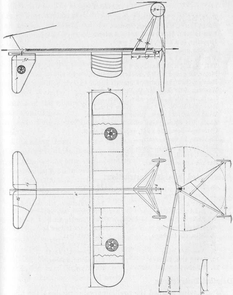
Fig. 79—3-Plan Drawing—Sky Flyer
