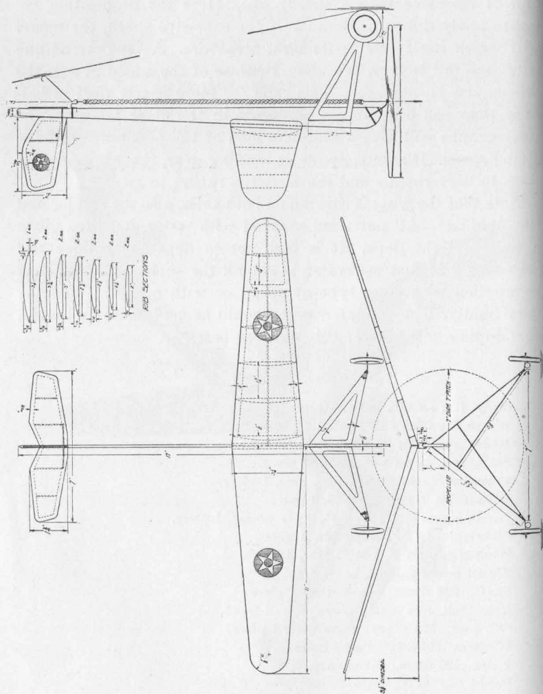
Fig. 82—3-Plan Drawing—Sky Raider
