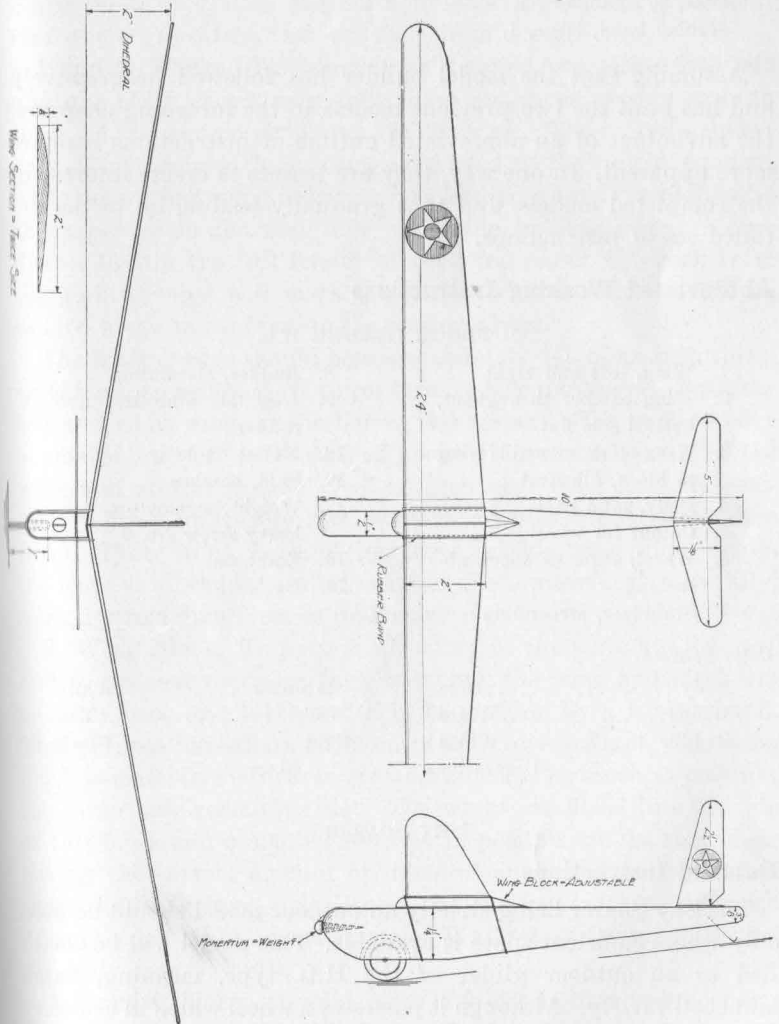
Fig. 73—3-Plan Drawing Sky Soarer
